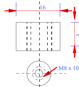
Złącze akumulatora
